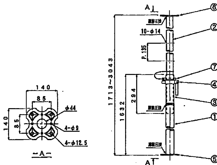
構造図
